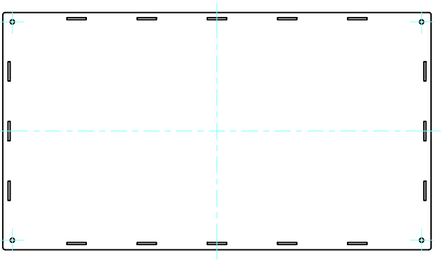
下カバー裏面 / Bottom cover Backside
