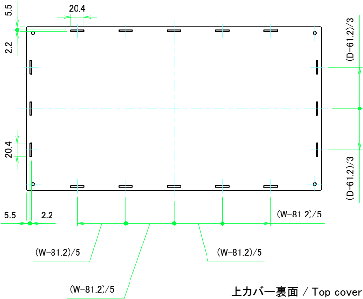
上カバー裏面 / Top cover Backside
