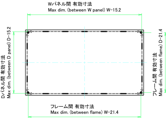
下カバー / Bottom cover
