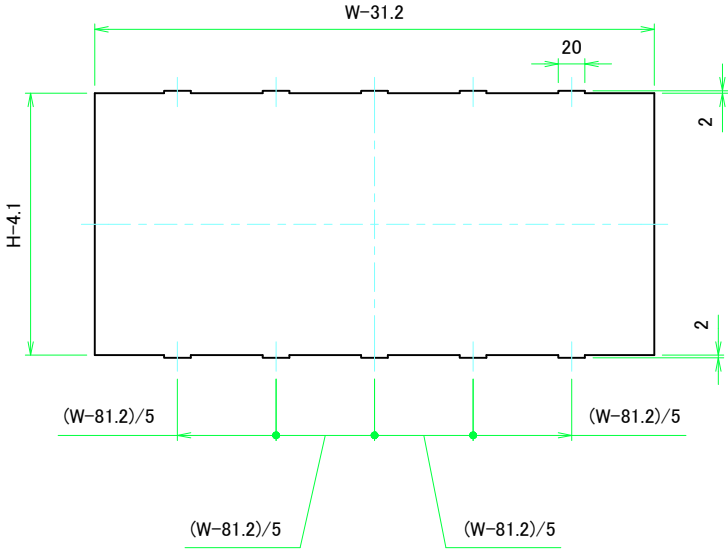
Wパネル1表面 / W Panel 1 Frontside
