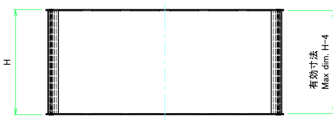
Wパネル1 / W Panel 1
